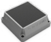
인증된 텅스텐 소재의 단파장 EMS 시준기
